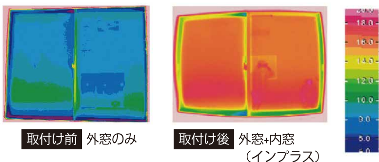
冬季における窓の室内側表面温度の比較
